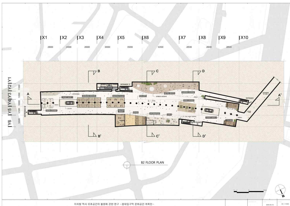
[그림 4-12] B2 FLOOR PLAN_ COLOR
