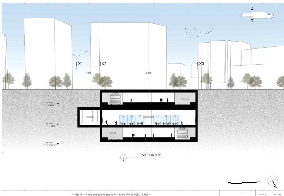
[그림 4-16] SECTION B-B'
