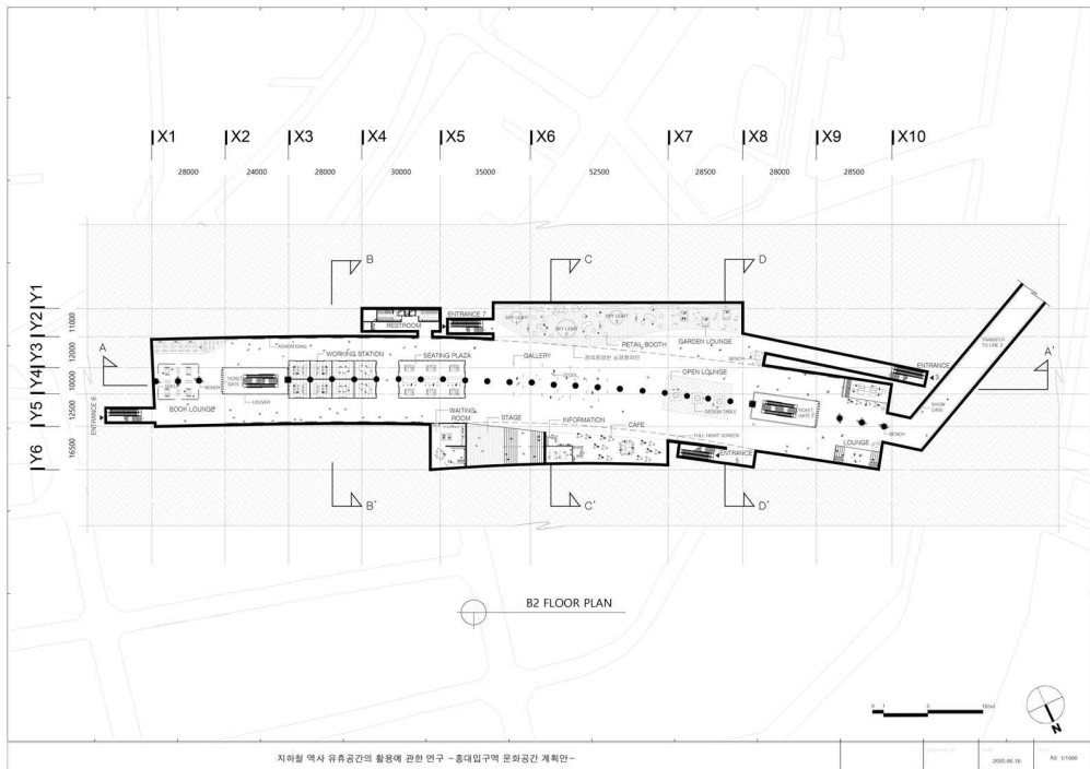
[그림 4-11] B2 FLOOR PLAN
