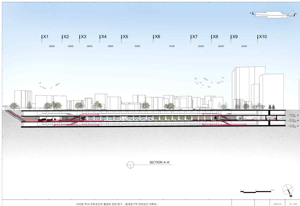
[그림 4-15] SECTION A-A'
