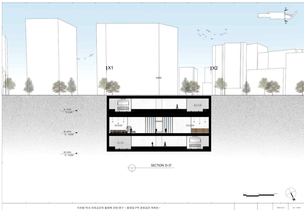
[그림 4-18] SECTION D-D'
