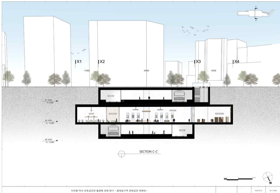
[그림 4-17] SECTION C-C'
